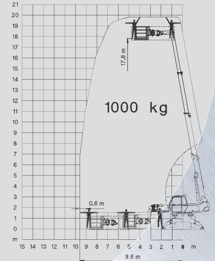
360° ABGESTÜTZT MIT ARBEITSBÜHNE VERSTELLBAR 1000 KG - 2/4 m
