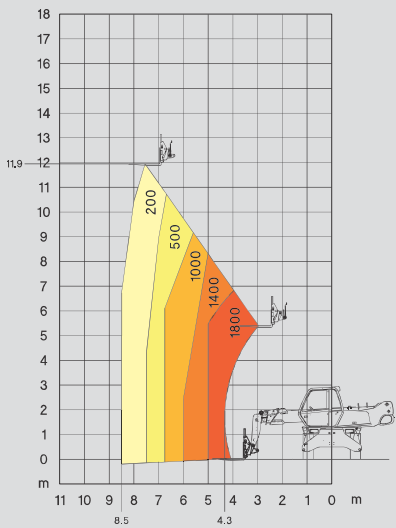
360° AUF REIFEN MIT GABELN
