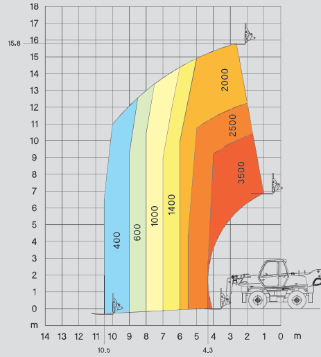
360° ABGESTÜTZT MIT SEILWINDE 3T
