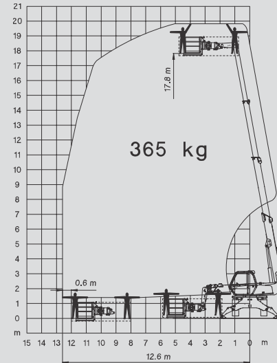
360° ABGESTÜTZT MIT ARBEITSBÜHNE VERSTELLBAR 365 KG - 2/4 m
