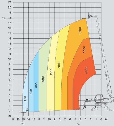
360° AUF REIFEN MIT GABELN
